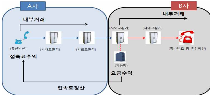
<A사 유선발신 B사 지능망 착신 예시>
